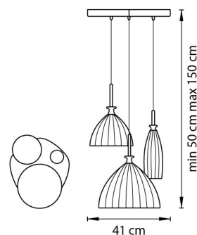
ЛЮСТРА ПОДВЕСНАЯ 3 x E14 max 40W 4,5 kg
