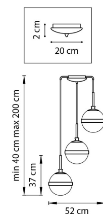
ЛЮСТРА ПОДВЕСНАЯ 3 x E14 max 40W 4 kg
