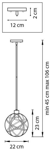
ЛЮСТРА ПОТОЛОЧНАЯ 1 x E27 max 40W 1,1 kg
