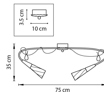
ЛЮСТРА ПОТОЛОЧНАЯ 6 x G9 max 25W / 6 x G9 LED 6W 2,6 kg
