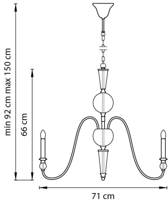
ЛЮСТРА ПОДВЕСНАЯ 6 x E14 max 40W 7,7 kg
