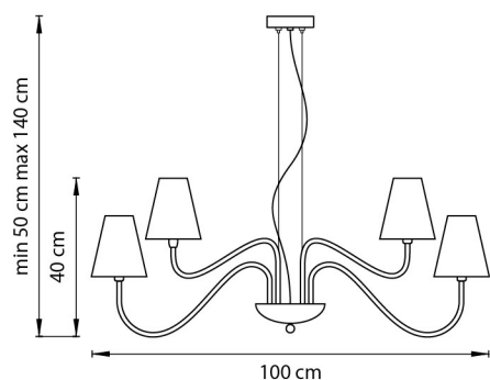
ЛЮСТРА ПОДВЕСНАЯ 16 x G9 max 40W 8 kg
