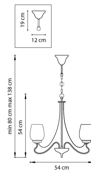
ЛЮСТРА ПОДВЕСНАЯ 5 x E14 max 40W 3,9 kg
