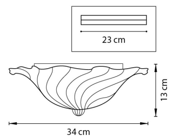
ЛЮСТРА ПОТОЛОЧНАЯ 3 x E14 max 40W 2 kg
