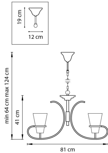
ЛЮСТРА ПОДВЕСНАЯ 6 x E14 max 40W 6,7 kg
