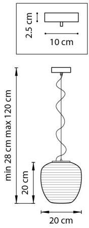
ЛЮСТРА ПОДВЕСНАЯ 1 x E27 max 40W 1,2 kg
