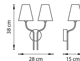
БРА 2 x G9 max 40W 0,8 kg
