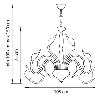
ЛЮСТРА ПОДВЕСНАЯ 24 x G4 12V max 20W 18,6 kg
