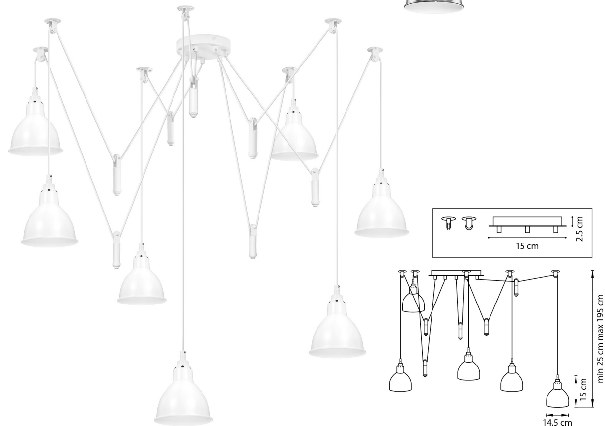
ЛЮСТРА ПОДВЕСНАЯ 7 x E14 max 40W 5,6 kg
