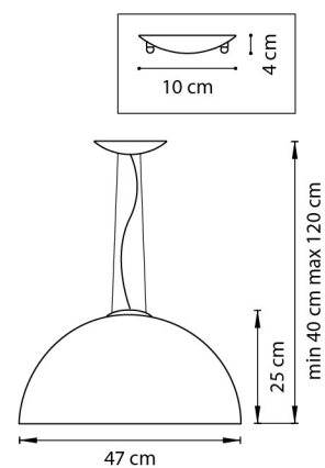
ЛЮСТРА ПОДВЕСНАЯ 1 x E27 max 40W 4,7 kg
