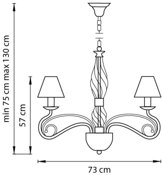
ЛЮСТРА ПОДВЕСНАЯ 8 x E14 max 40W 5,5 kg
