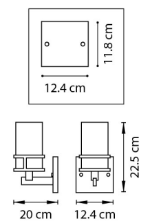
БРА 1 x E14 max 40W 0,9 kg
