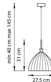
ЛЮСТРА ПОДВЕСНАЯ 1 x E14 max 40W 2,2 kg
