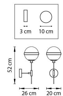
БРА 1 x E14 max 40W 1,8 kg
