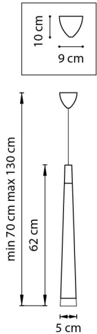
ЛЮСТРА ПОДВЕСНАЯ 1 x G9 max 25W / 1 x G9 LED 6W 0,7 kg
