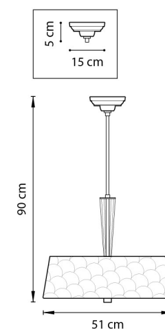
ЛЮСТРА ПОТОЛОЧНАЯ 6 x E14 max 40W 5,6 kg
