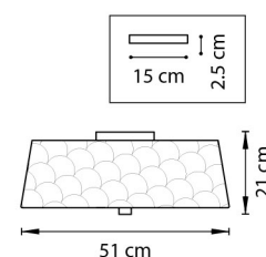
ЛЮСТРА ПОТОЛОЧНАЯ 6 x E14 max 40W 4,3 kg
