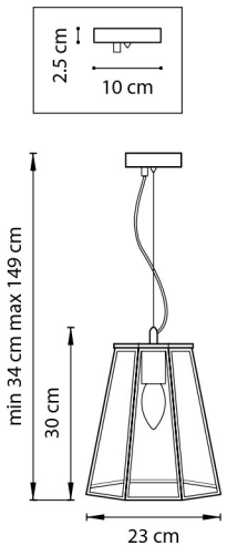
ЛЮСТРА ПОДВЕСНАЯ 1 x E27 max 40W 1,6 kg
