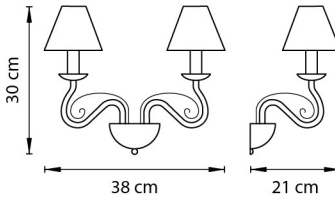
БРА 2 x E14 max 40W 1,2 kg
