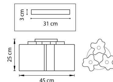
ЛЮСТРА ПОТОЛОЧНАЯ 3 x E27 max 40W 4,3 kg
