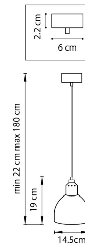
ЛЮСТРА ПОДВЕСНАЯ 1 x E14 max 40W 0,5 kg
