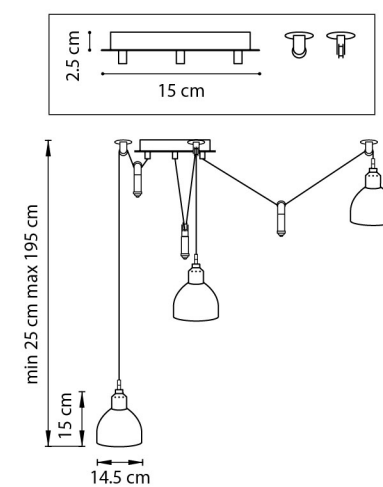
ЛЮСТРА ПОДВЕСНАЯ 5 x E14 max 40W 4 kg
