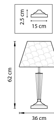
НАСТОЛЬНАЯ ЛАМПА 1 x E14 max 40W 3,3 kg
