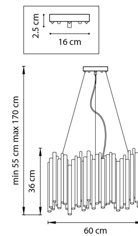
ЛЮСТРА ПОДВЕСНАЯ 10 x G9 max 40W 8,3 kg
