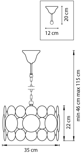
ЛЮСТРА ПОДВЕСНАЯ 4 x E14 max 40W 3,3 kg
