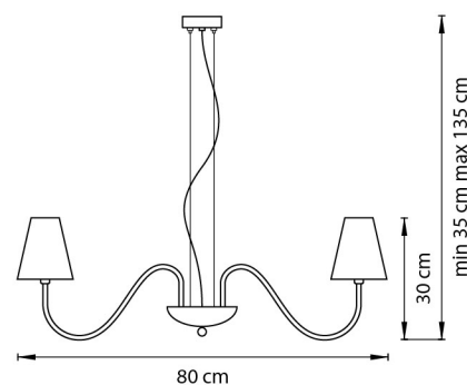
ЛЮСТРА ПОДВЕСНАЯ 8 x G9 max 40W 758082 4 kg 758084 3 kg
